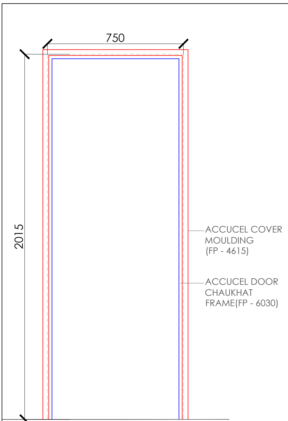
FRAME ELEVATION
